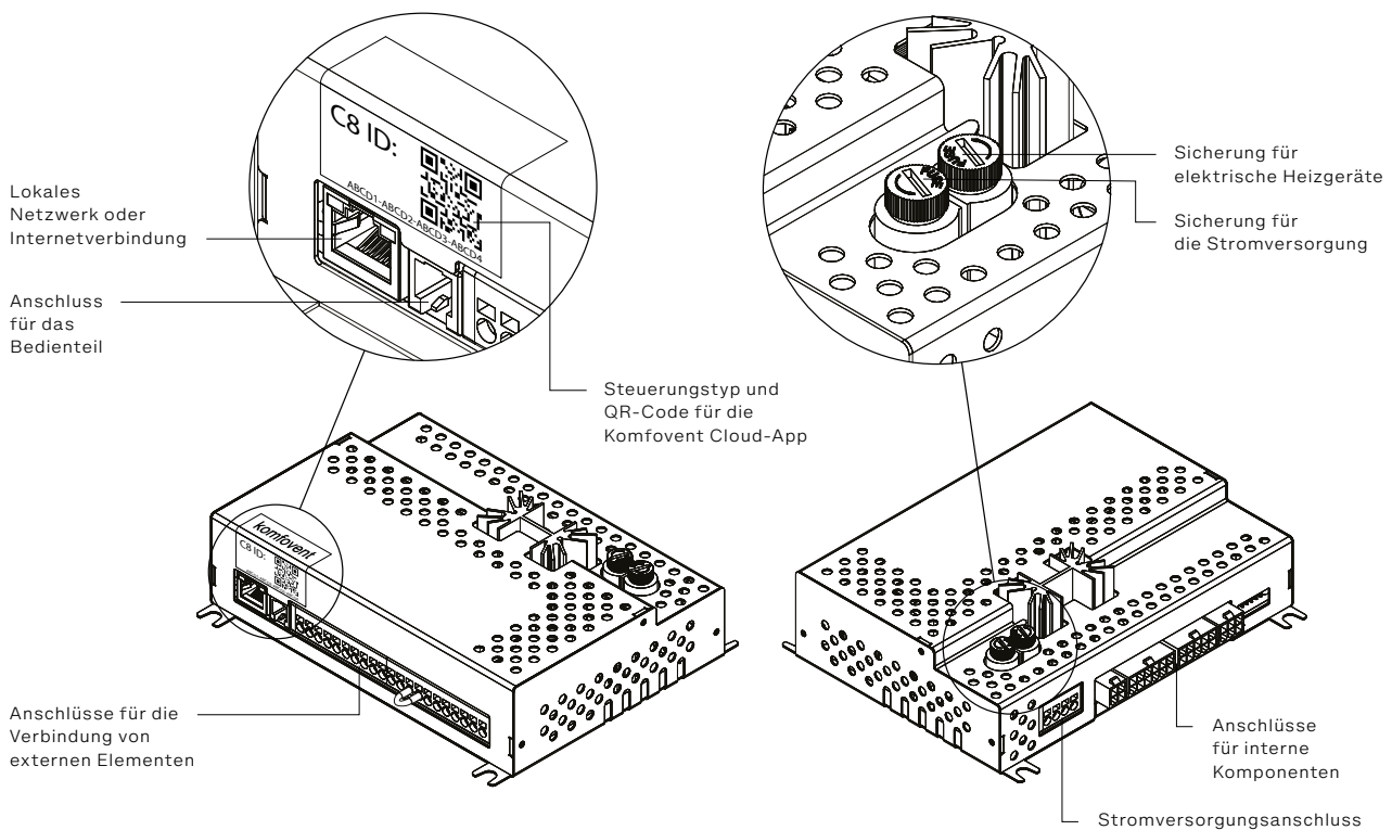
Abb. C8 Steuerung-Hauptboard
